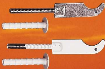
Wieszak grzejnikowy z kolkiem ocynk lub biały
